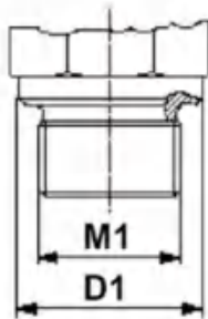
DIN3852-1 形式B ISO1179-3 硬密封结构
