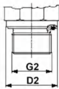
DIN3852-11 形式E IS01179-2 带弹性体密封结构
