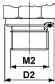
DIN3852-11 形式E ISO9974-2 带弹性体密封结构
